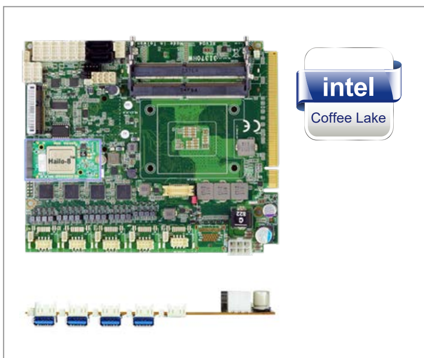
3I370HW + Hailo-8™ AI module
