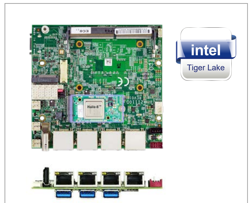
2I110D + Hailo-8™ AI module
