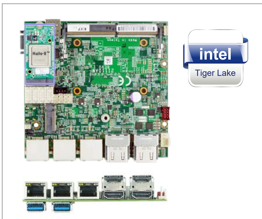
2I110AW + Hailo-8™ AI module
