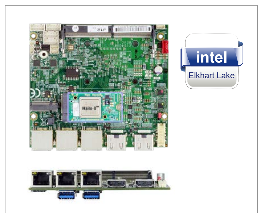
2I640DW + Hailo-8™ AI module
