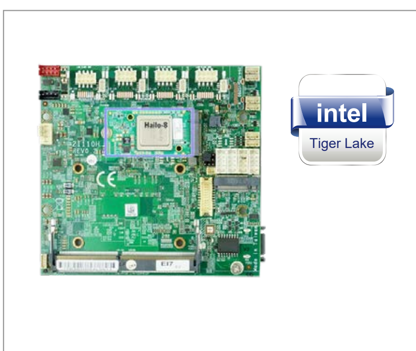
2I110H + Hailo-8™ AI module
